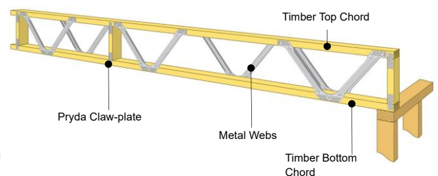
SPACEJOIST™ TRUSS
